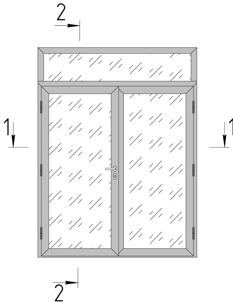
Дверь двустворчатая с фрамугой
