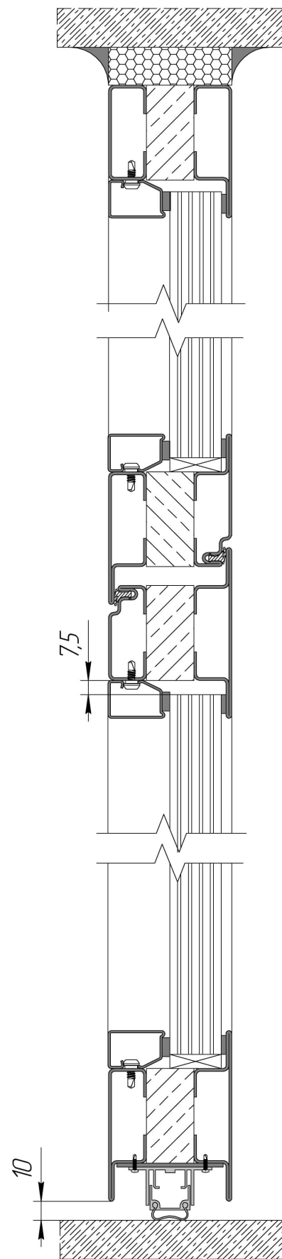
Вариант 2 С выпадющим порогом
